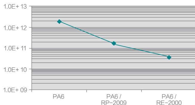
图二：降低材料电阻 \Omega - ISO 10965
