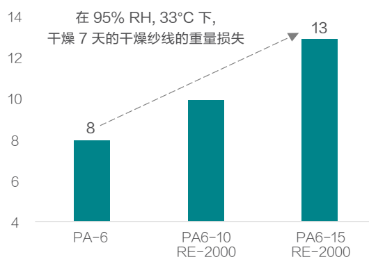
图一：锦纶纤维吸湿性，%
